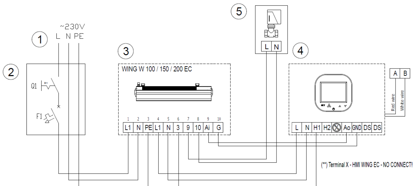
Przykładowy schemat podłączenia kurtyzny WING W100-200 EC, pełne schematy elektryczne dostępne do pobrania na www.vtsgroup.com Example connection diagram of WING W100-200 EC, full electrical diagrams available for download at www.vtsgroup.com .
